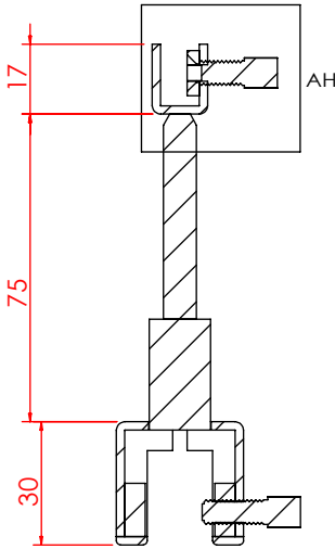
剖面 AG-AG
