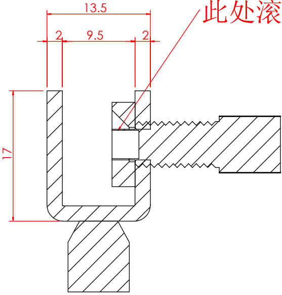
局部视图 AH 比例 2 : 1
