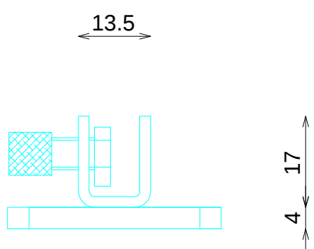
PERFIL
