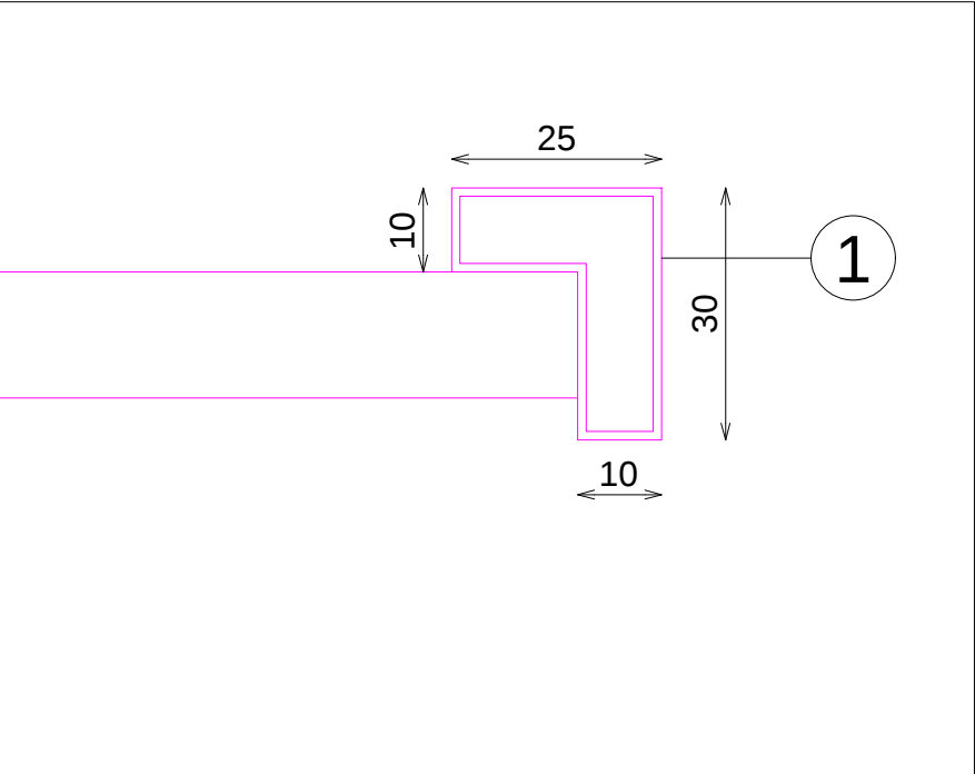
DETALLE BARRA ANCLAJE A PARED
