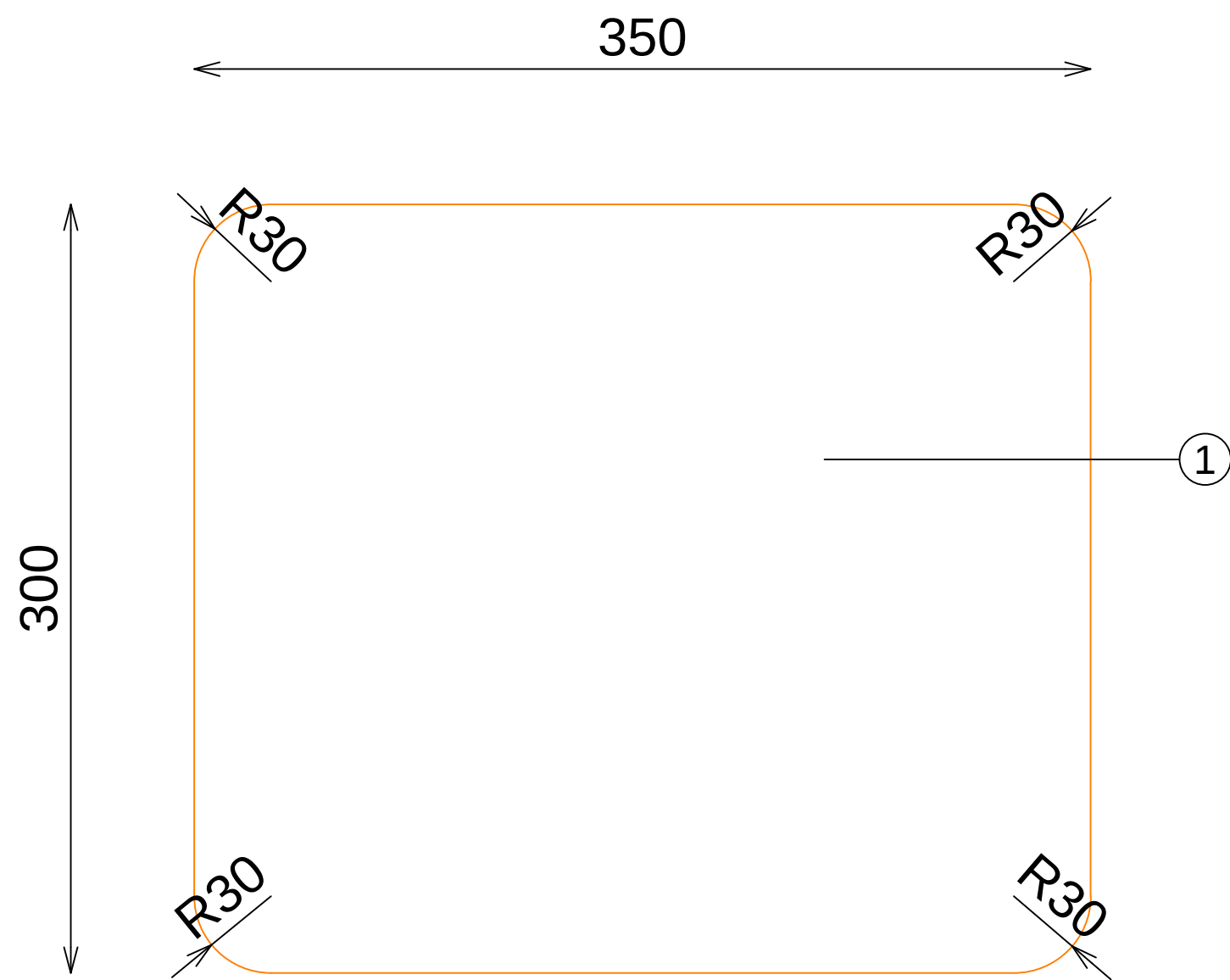
PLANTA
