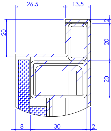
局部视图 B 比例 1 : 1
