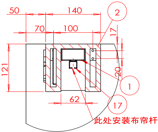
局部视图 D
