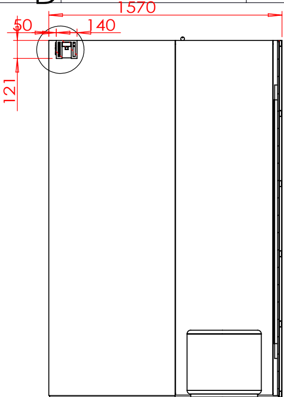
剖面 C-C
