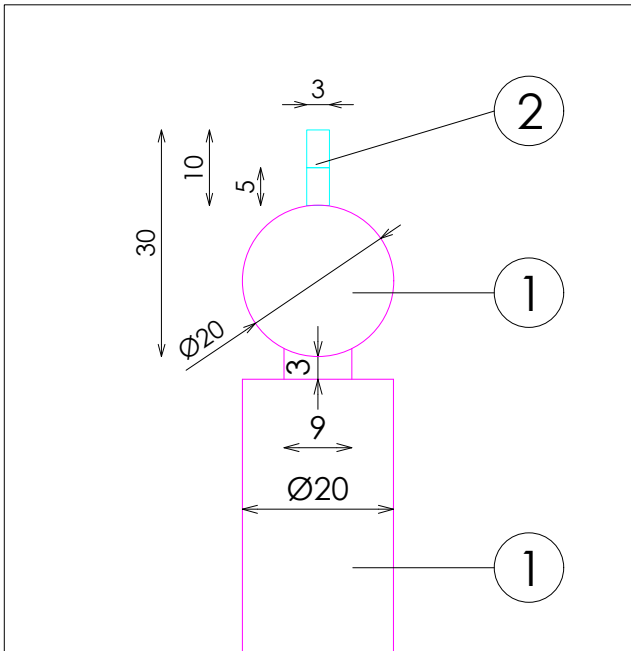
DETALLE ANTIROCE
