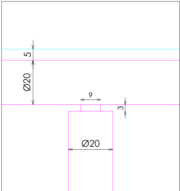
DETALLE C
