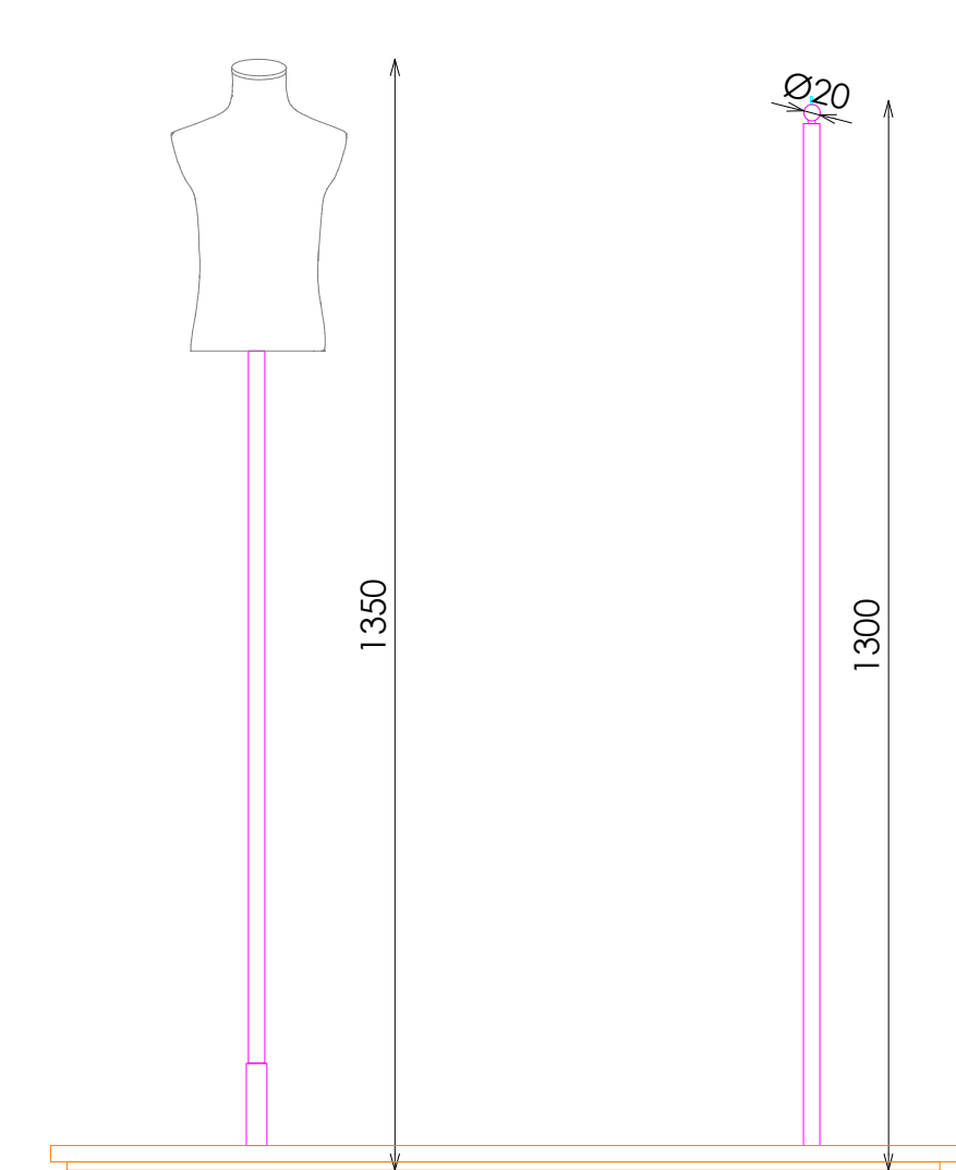
ALZADO
