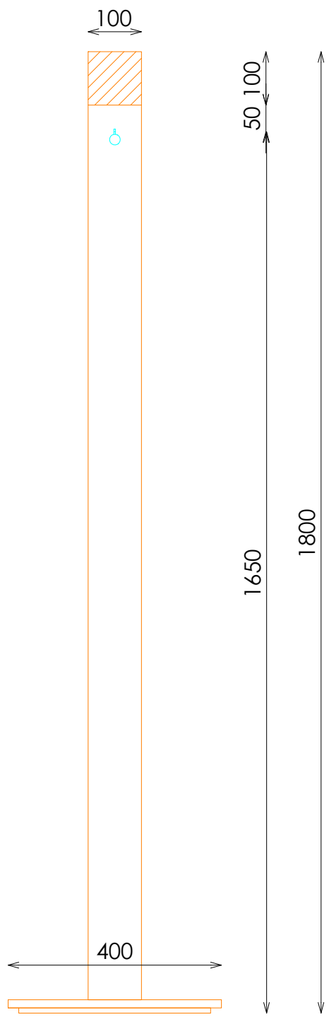
SECCION
