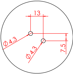
局部视图 AG 比例 1 : 2
