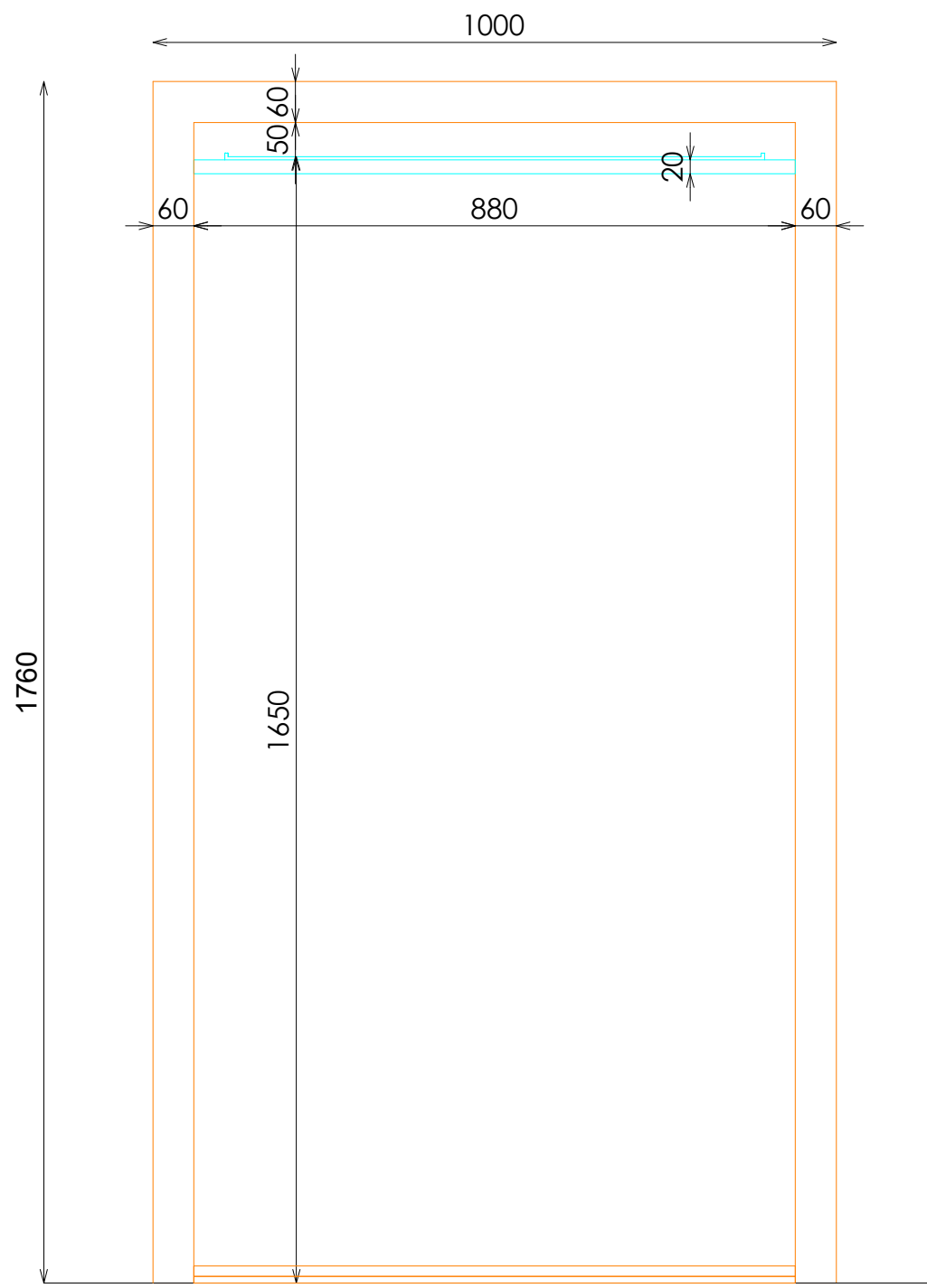
ALZADO
