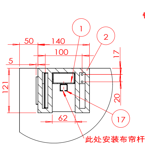
剖面 C-C
