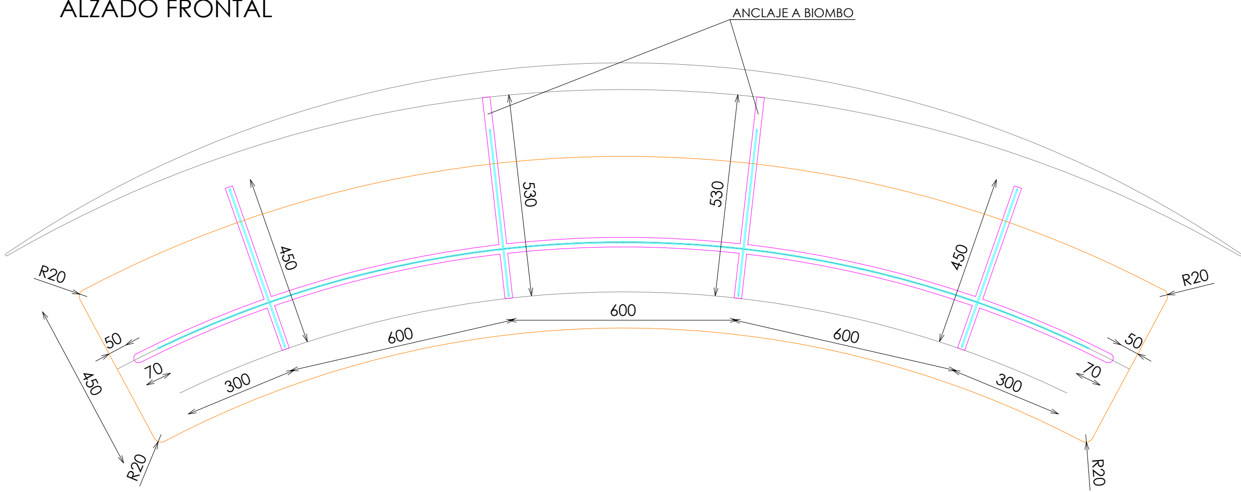
PLANTA BARRA
