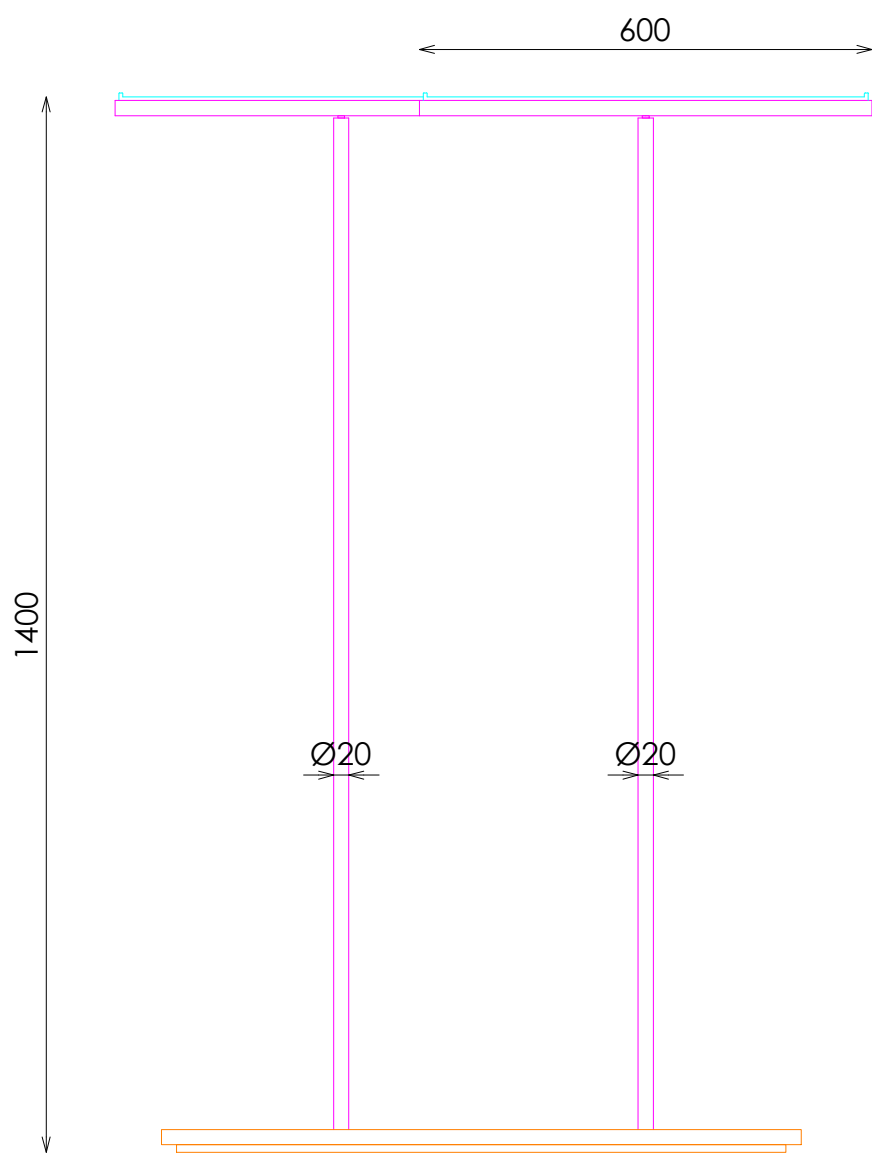
PERFIL DERECHO
