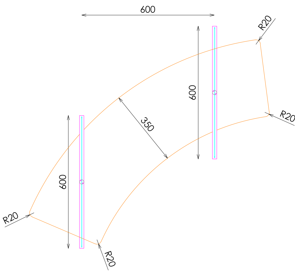
PLANTA
