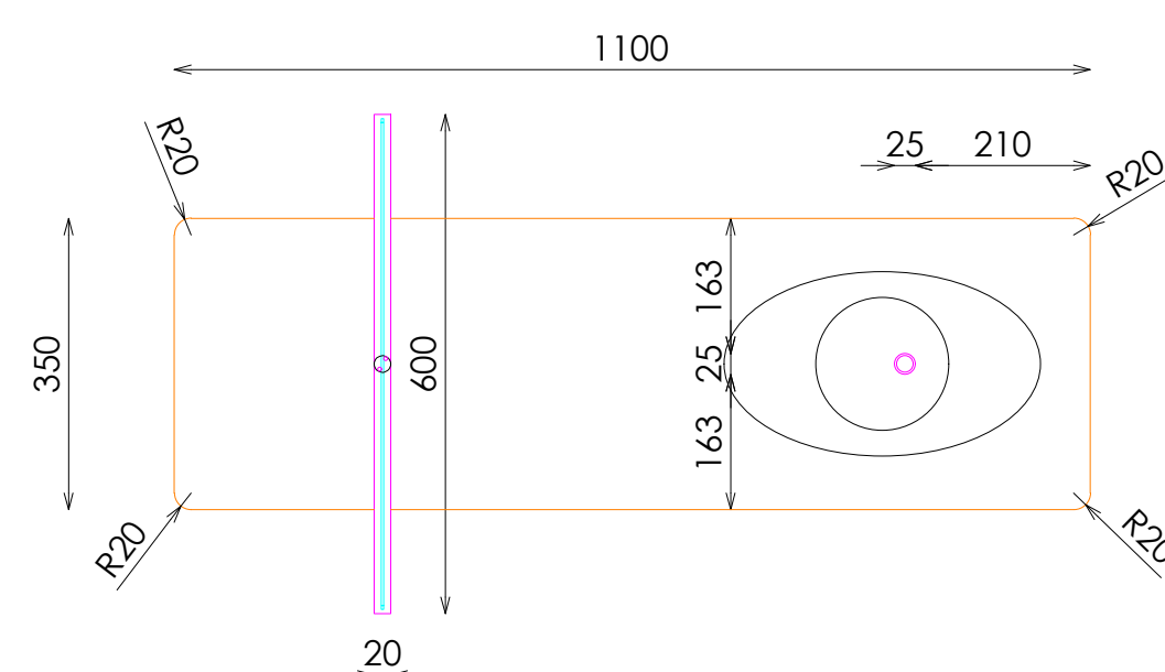
PLANTA
