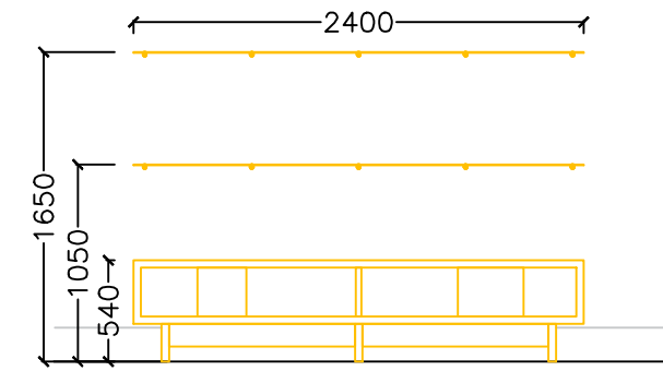
ALZADO ELEVATION
