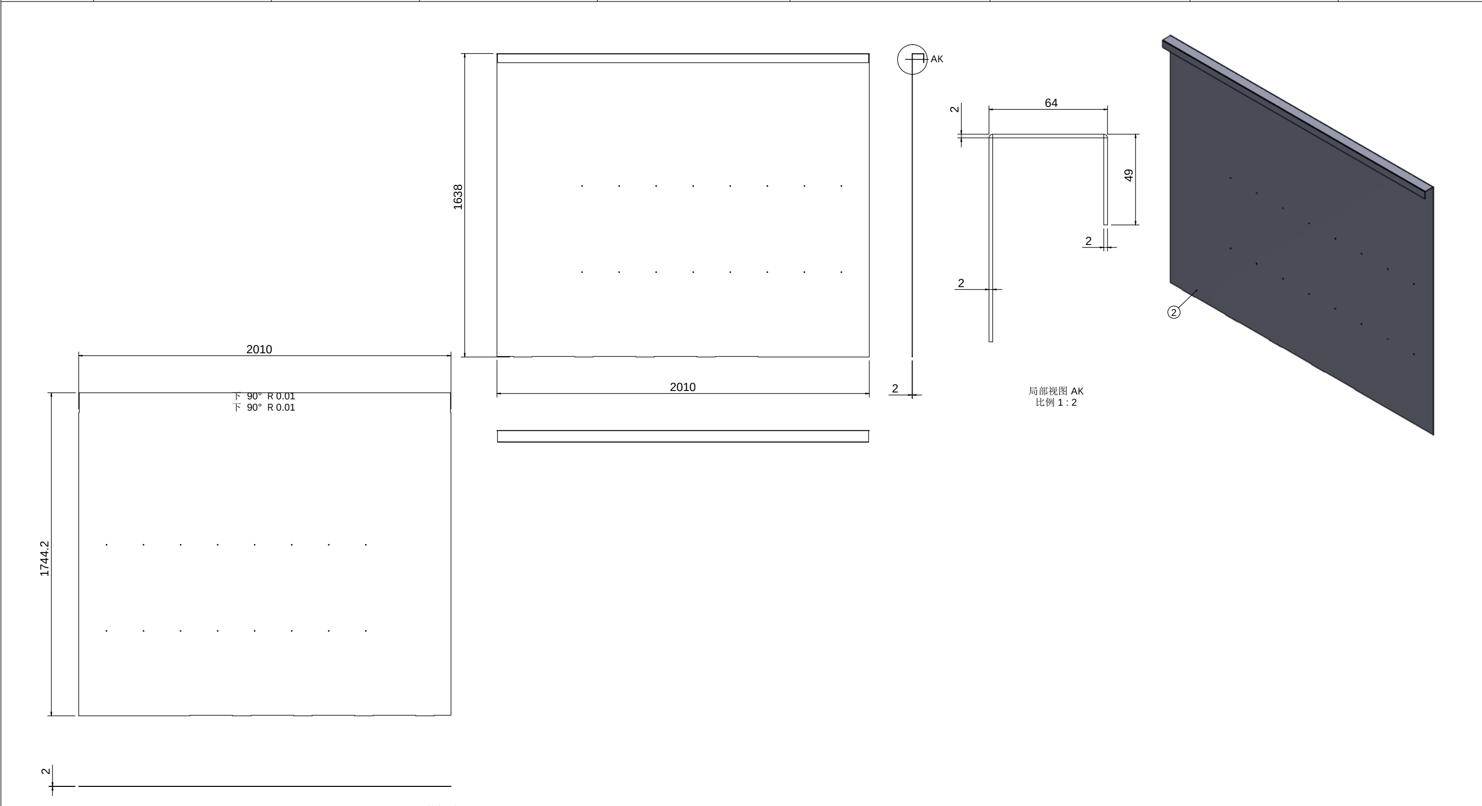
金属展开图
