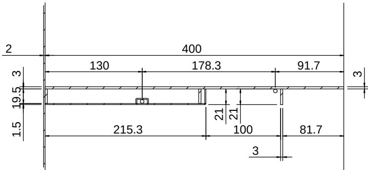
局部视图 AL 比例 1 : 5
