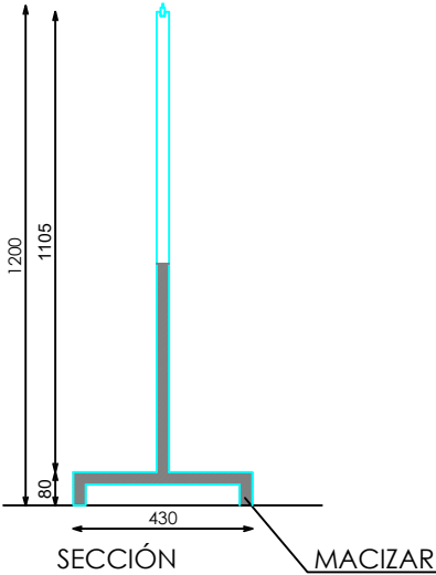
SECCIÓN
