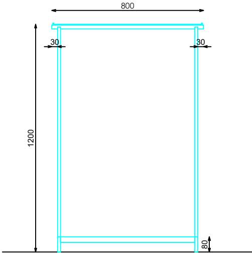
ALZADO
