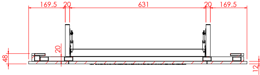
剖面 AH-AH 比例 1 : 10
