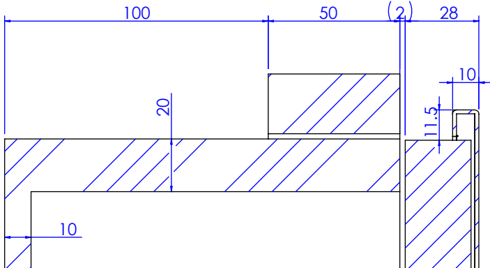
局部视图 AH 比例 1 : 2
