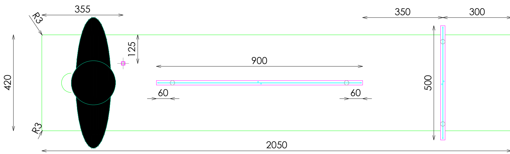
PLANTA
