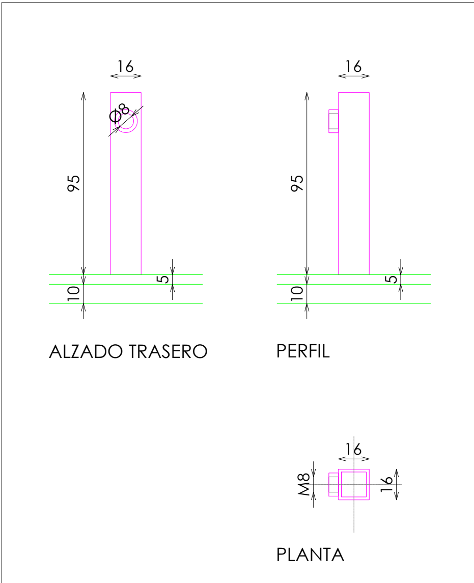
DETALLE ANCLAJE MANIQUI
