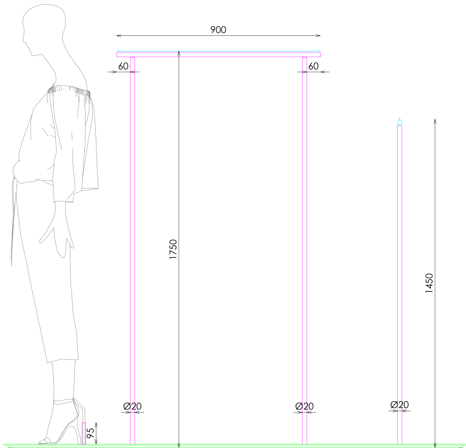
ALZADO LATERAL
