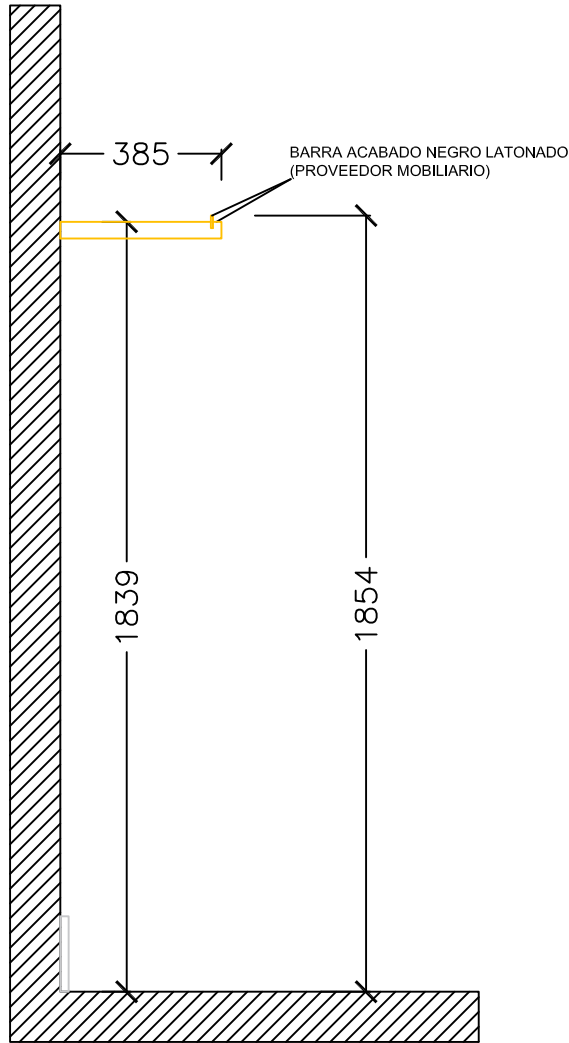
PERFIL SIDE ELEVATION
