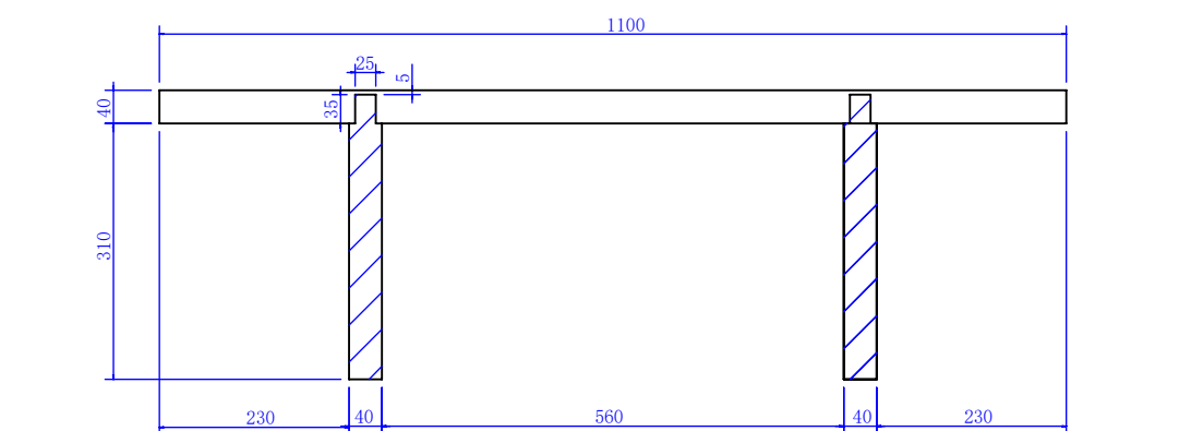
剖面 B-B
