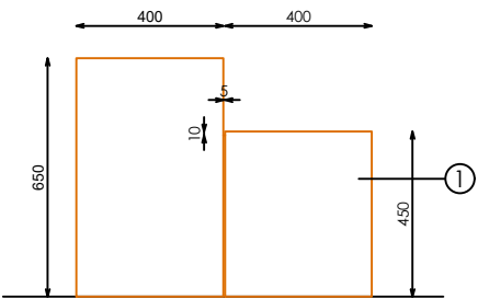
PERFIL
