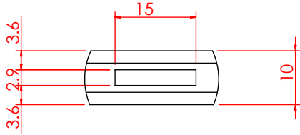
局部视图 AN 比例 1 : 1
