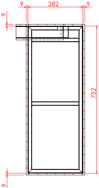
剖面 AI-AI 比例 1 : 10
