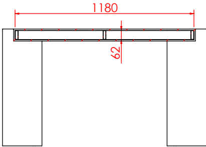
剖面 AH-AH
