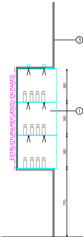
SECCIÓN
