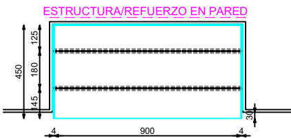
PLANTA
