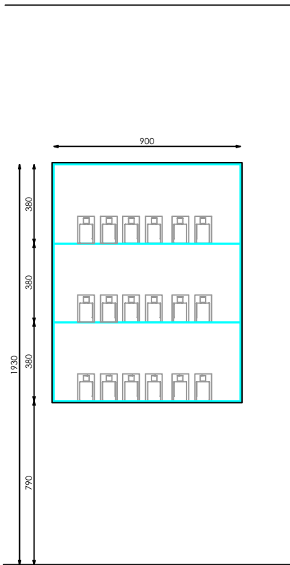
ALZADO FRONTAL
