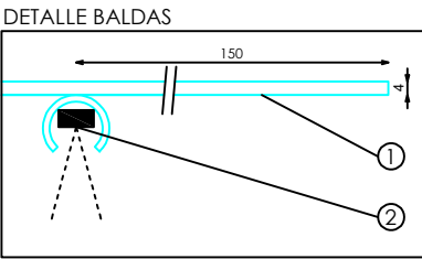
DETALLE BALDAS
