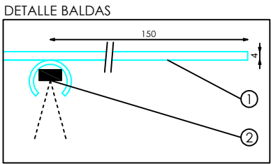
DETALLE BALDAS
