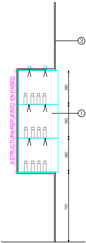
SECCIÓN
