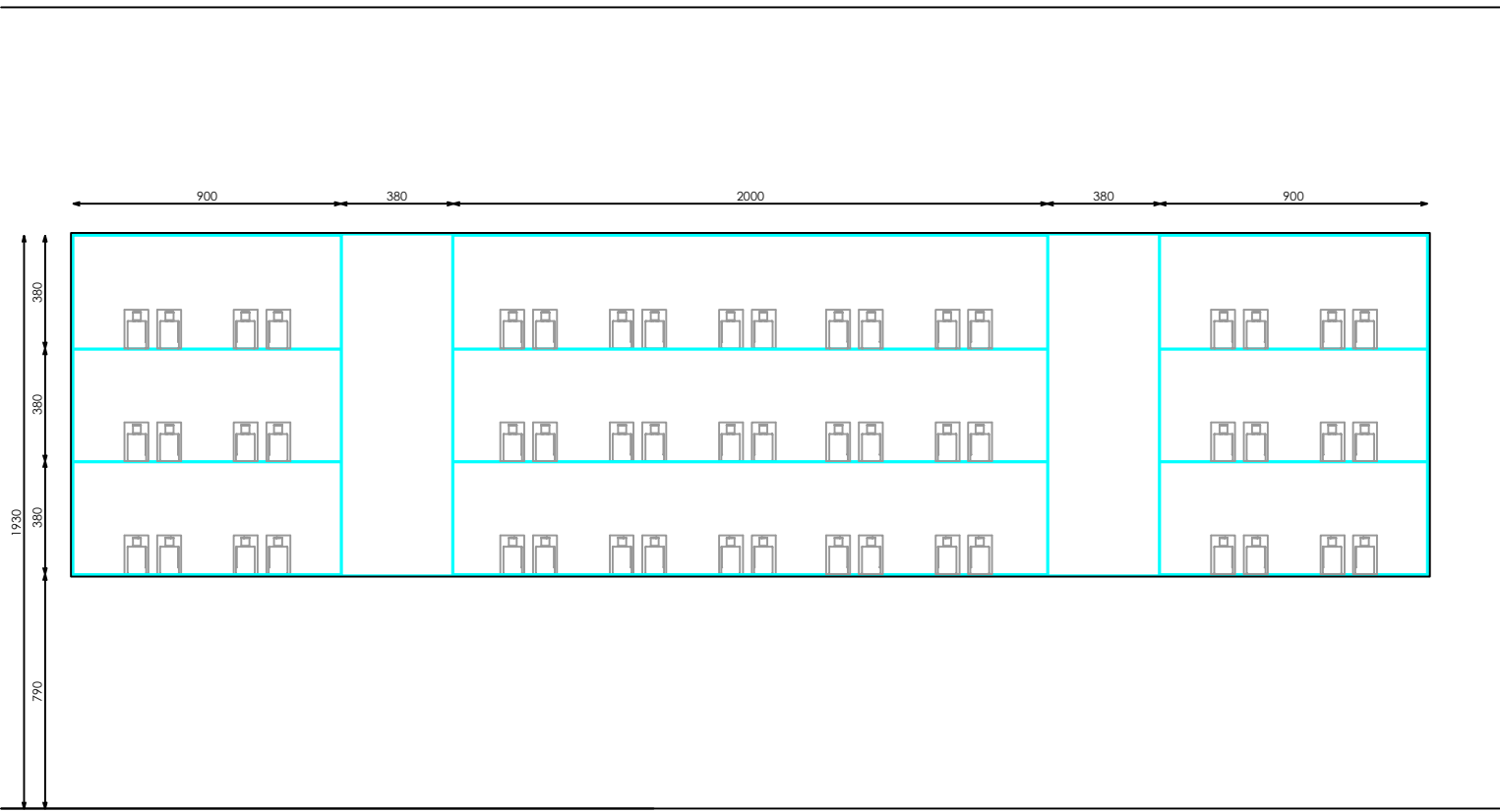
ALZADO FRONTAL
