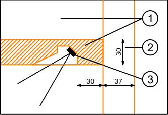
DETALLE ILUMINACION BALDA
