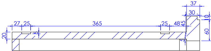
局部视图 AH 比例 1 : 5
