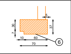
DETALLE REMATE IZQ.
