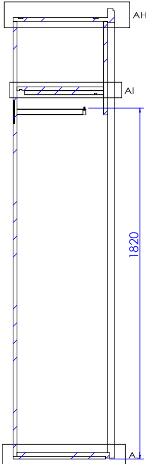
剖面 AG-AG
