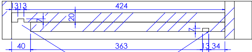
局部视图 AI 比例 1 : 5
