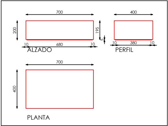
DETALLE MODULO 70x40xH20 (1 UNIDAD)
