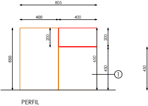
DETALLE MODULO 70x40xH20 (1 UNIDAD)
