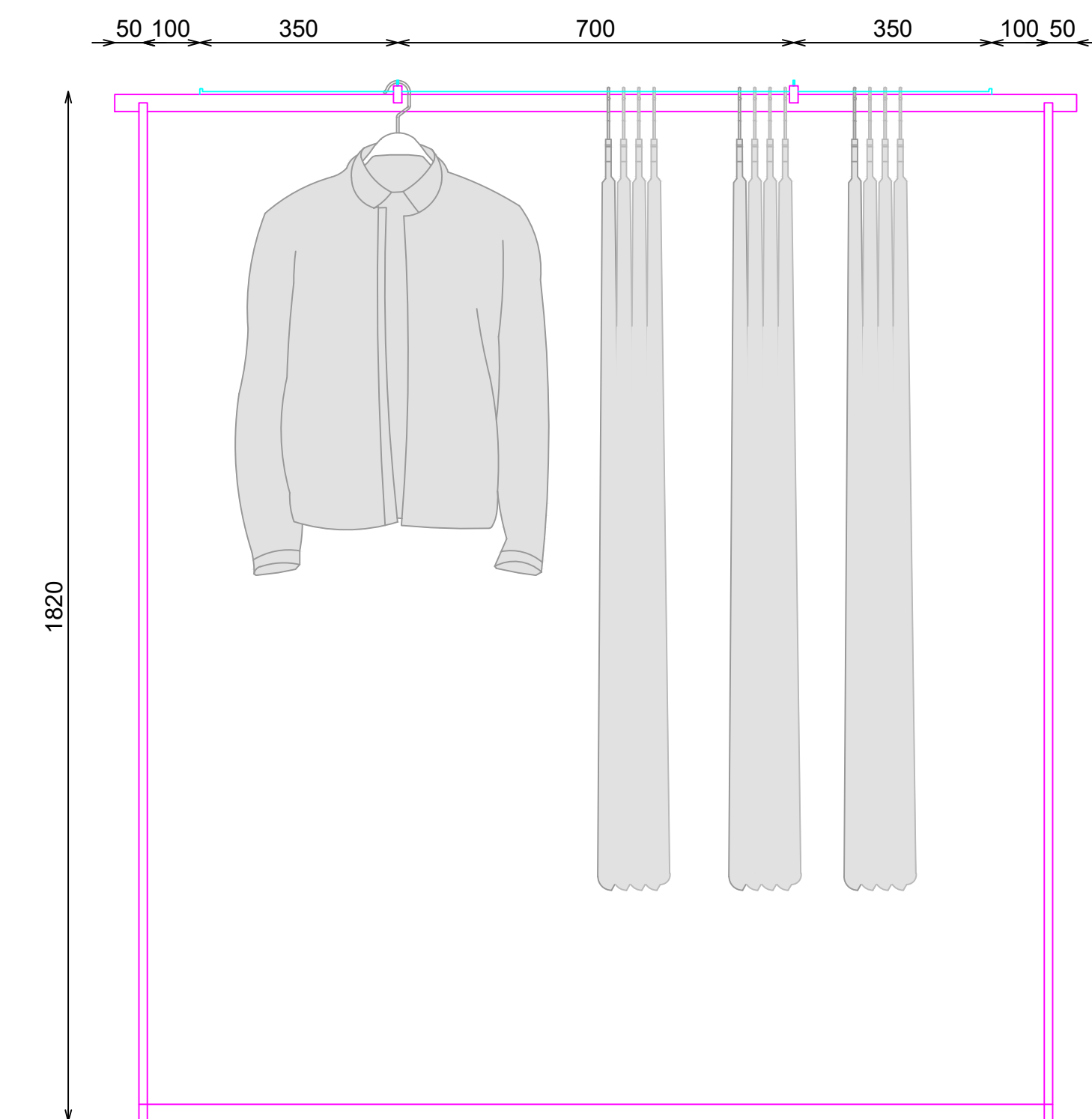
ALZADO
