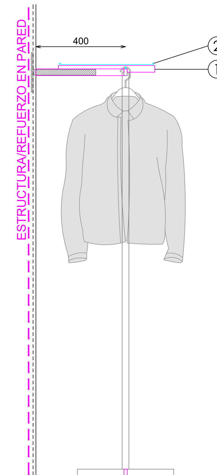
SECCION
