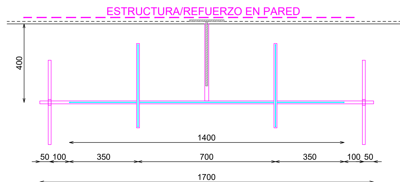
PLANTA
