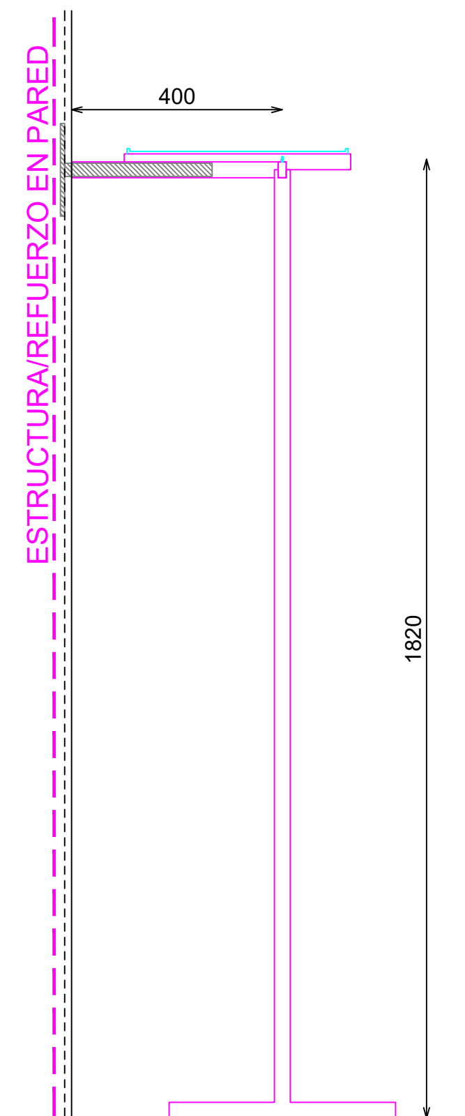
SECCION
