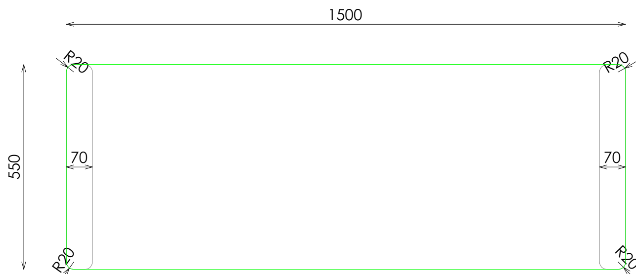
PLANTA MESA SECCIONADA
