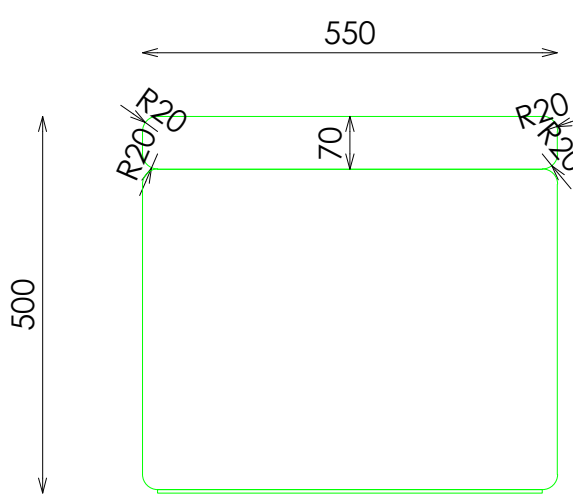
PERFIL
