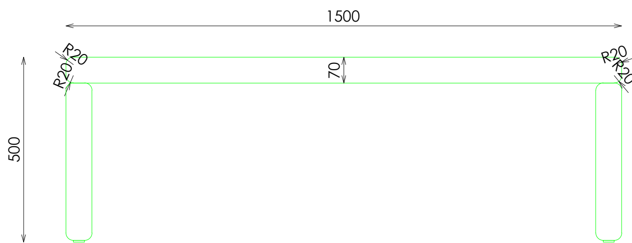
ALZADO
