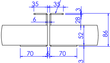
局部视图 AG 比例 1:5
