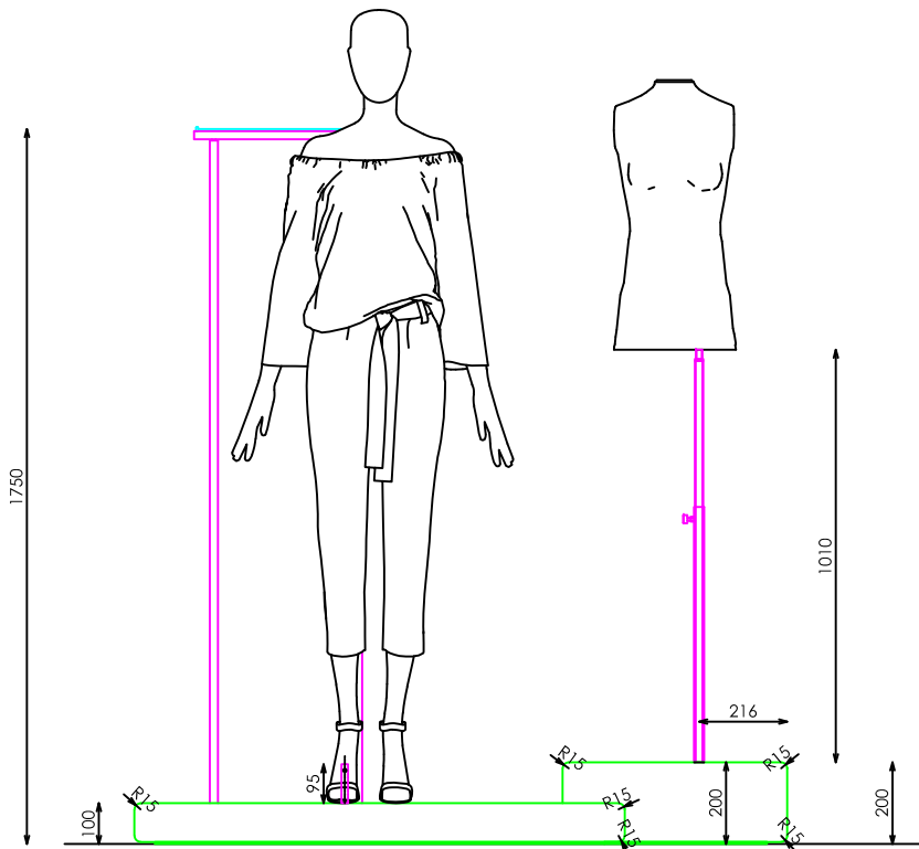
ALZADO FRONTAL
