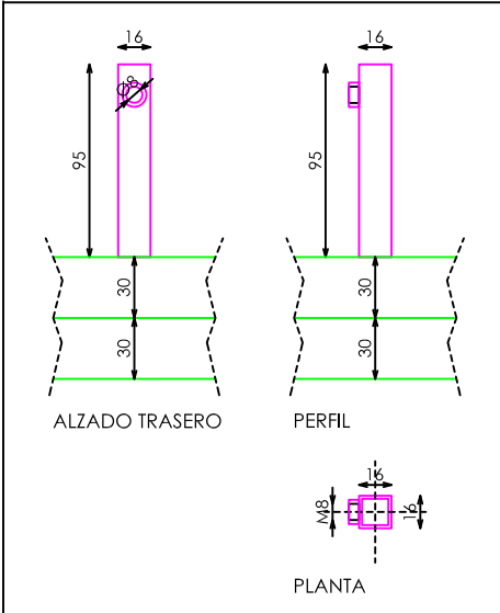
DETALLE ANCLAJE MANIQUI
