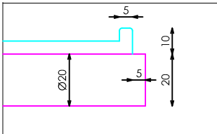
DETALLE ANCLAJE MANIQUI
