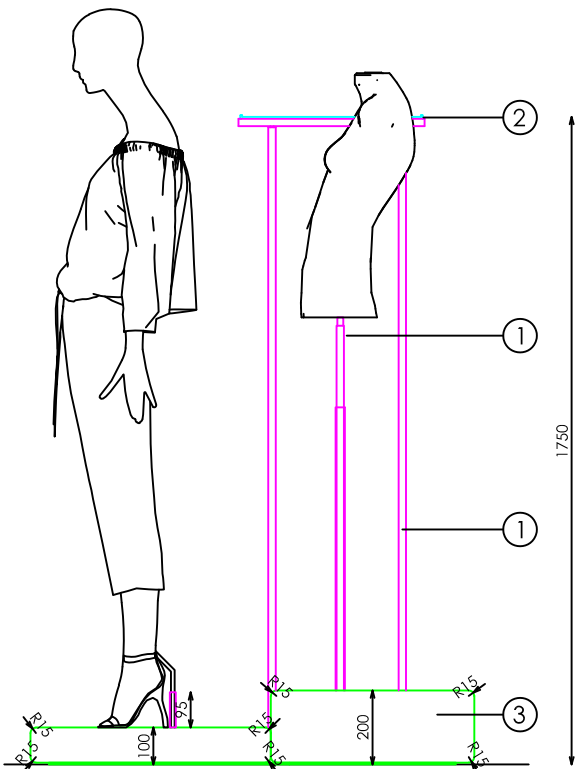
ALZADO LATERAL DERECHO
