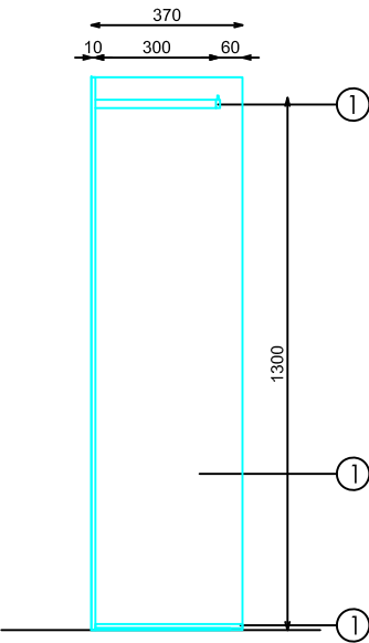
PERFIL
