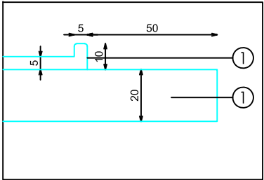
DETALLE B
