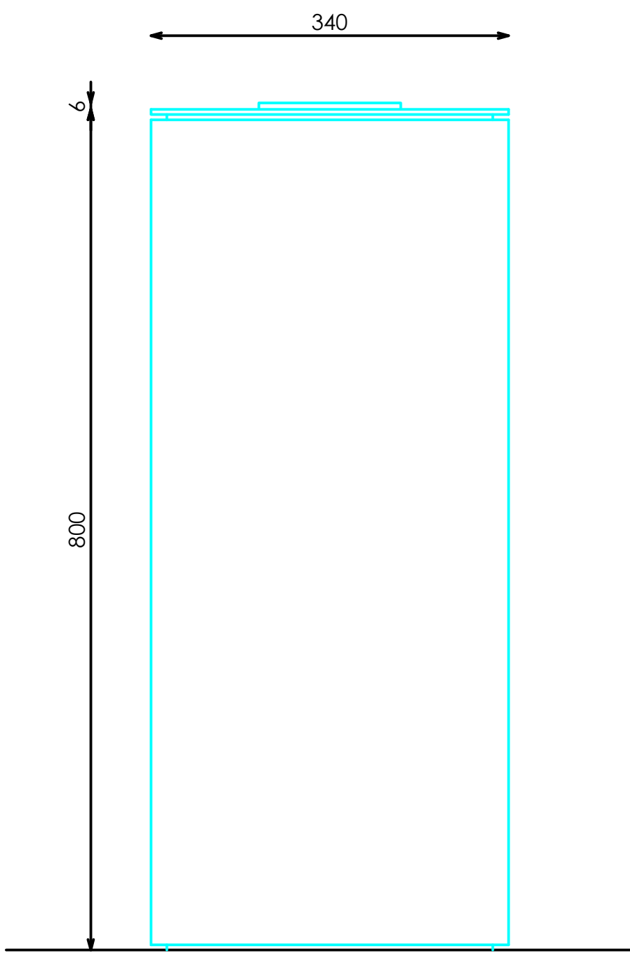
ALZADO LATERAL
