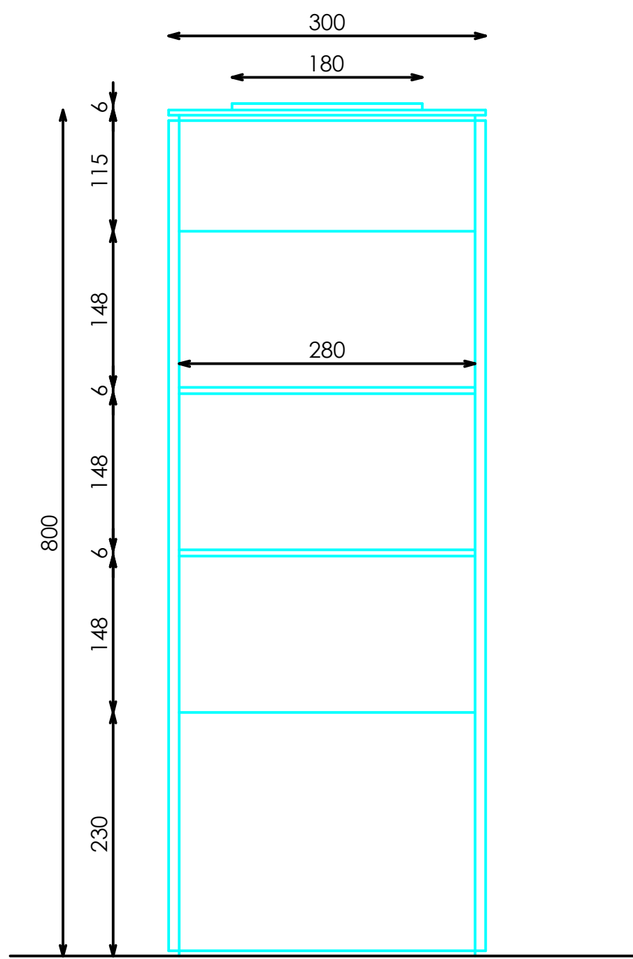
ALZADO FRONTAL
