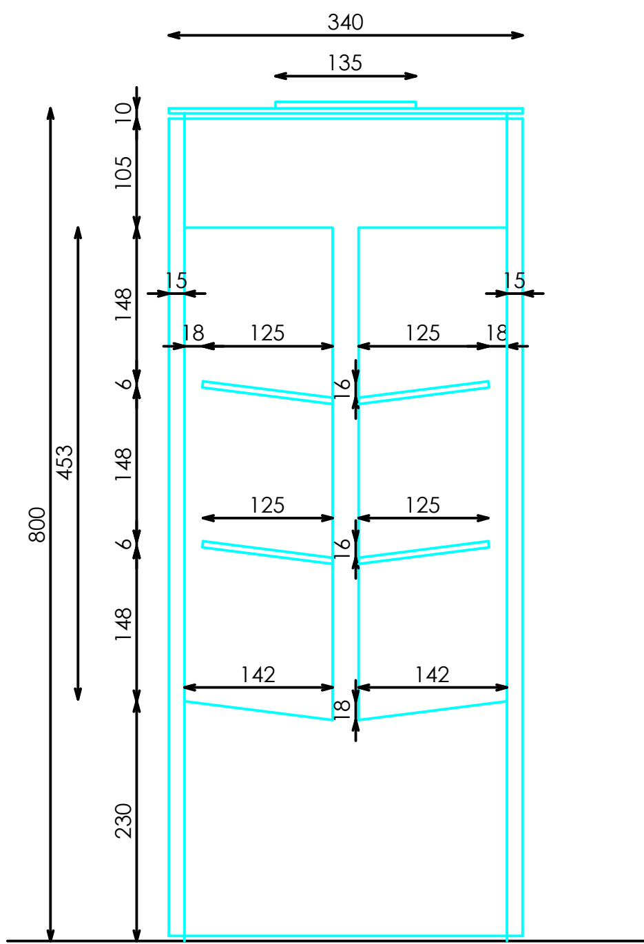
SECCION
