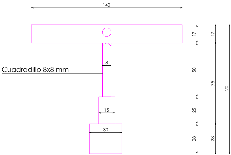
ALZADO
