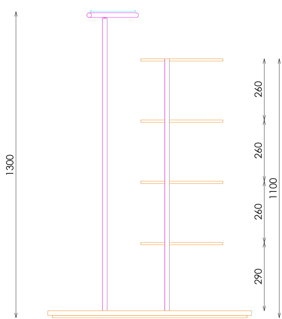
ALZADO
