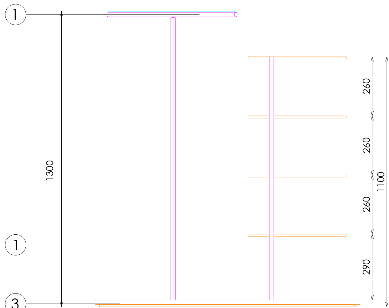
PERFIL DERECHO
