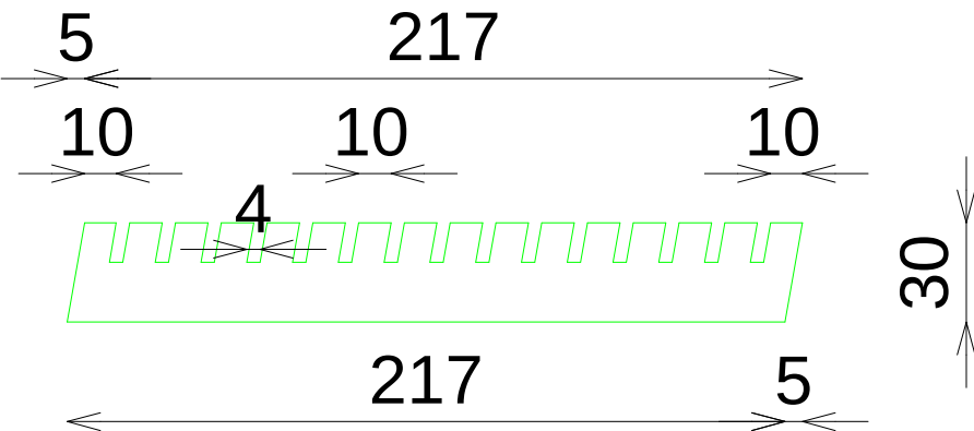
ALZADO
