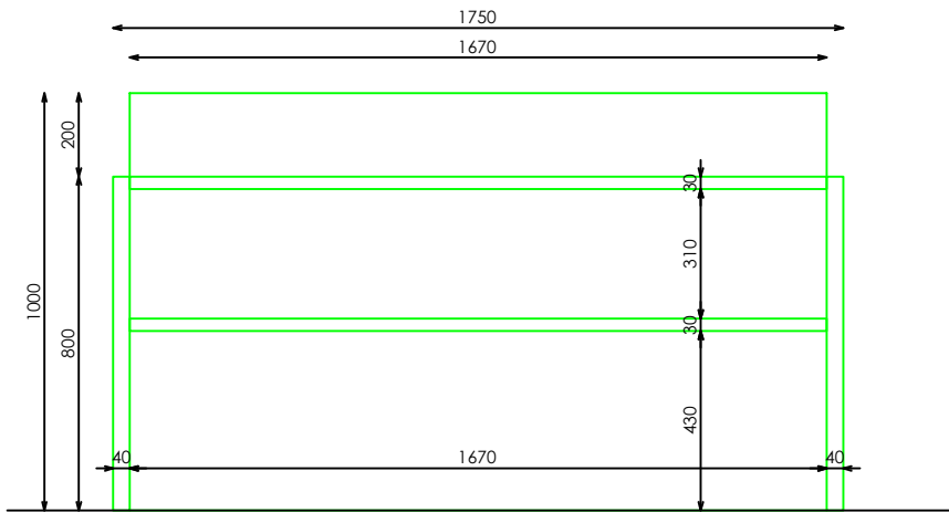
ALZADO FRONTAL
