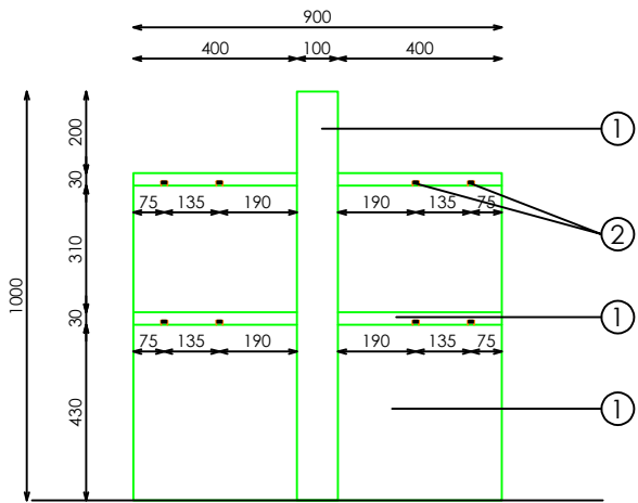
SECCION
