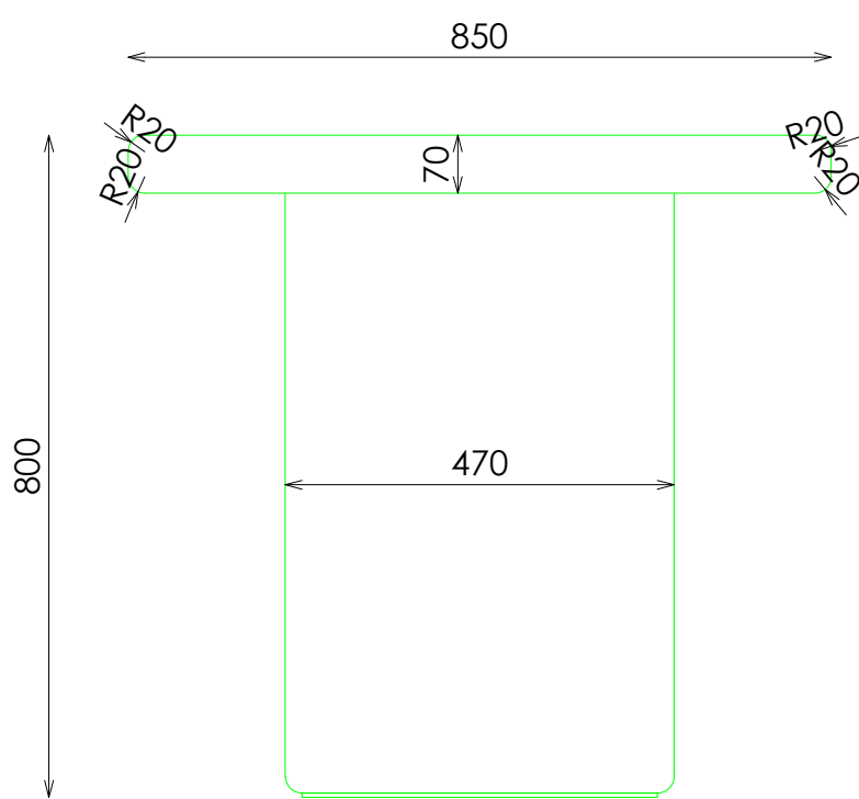
PERFIL
