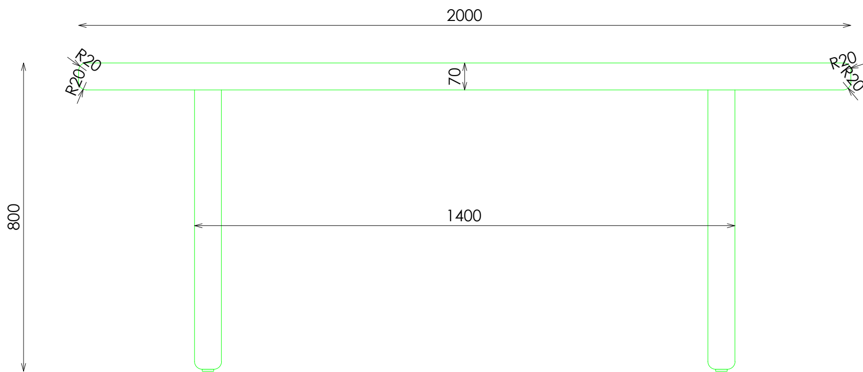
ALZADO
