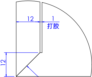
局部视图 AG 比例 1 : 1
