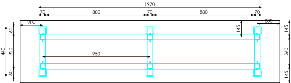
PLANTA SECCIONADA
