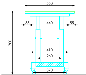
ALZADO LATERAL
