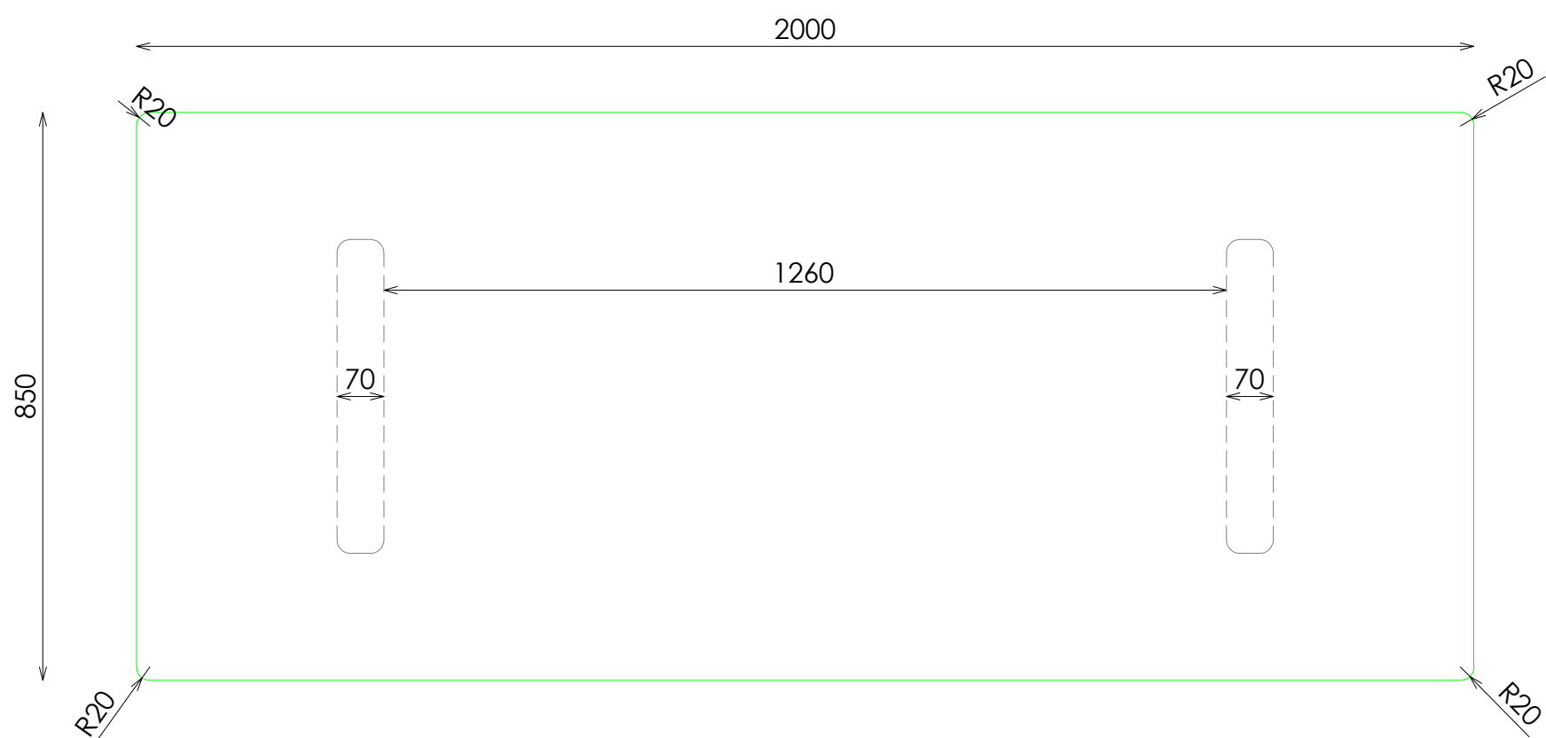
PLANTA
