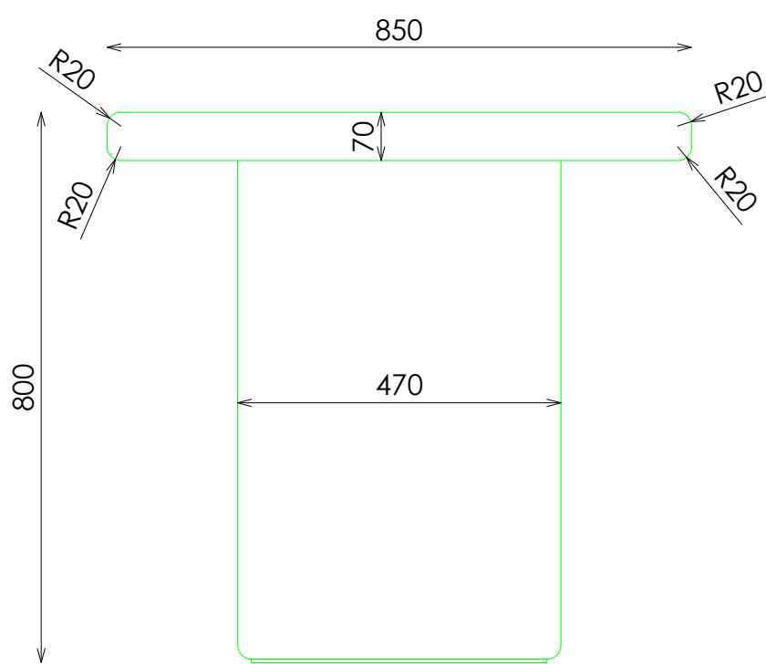
PERFIL
