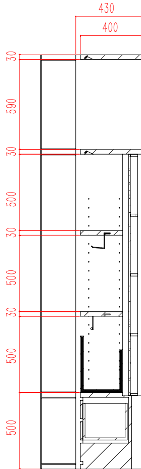
剖面 G-G
