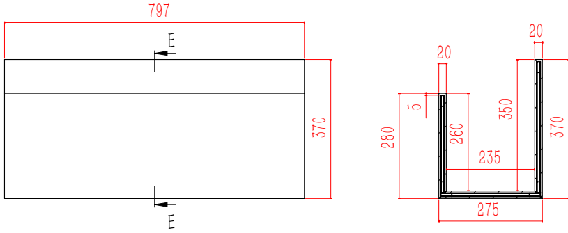
剖面 E-E
