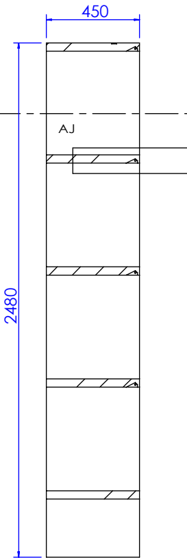
剖面 AH-AH
