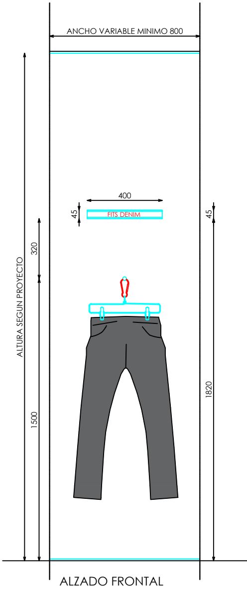
ALZADO FRONTAL
