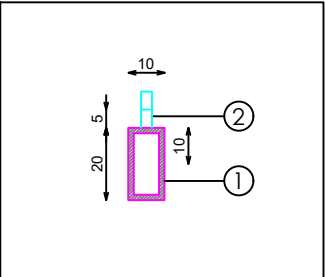
DETALLE A
