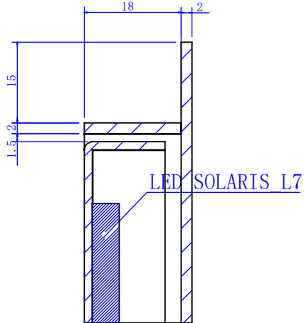
局部视图 B 比例 1 : 1
