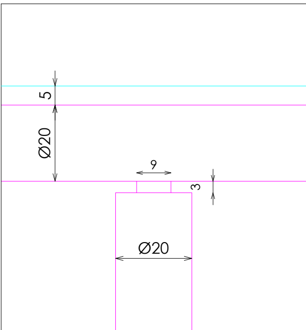
DETALLE C
