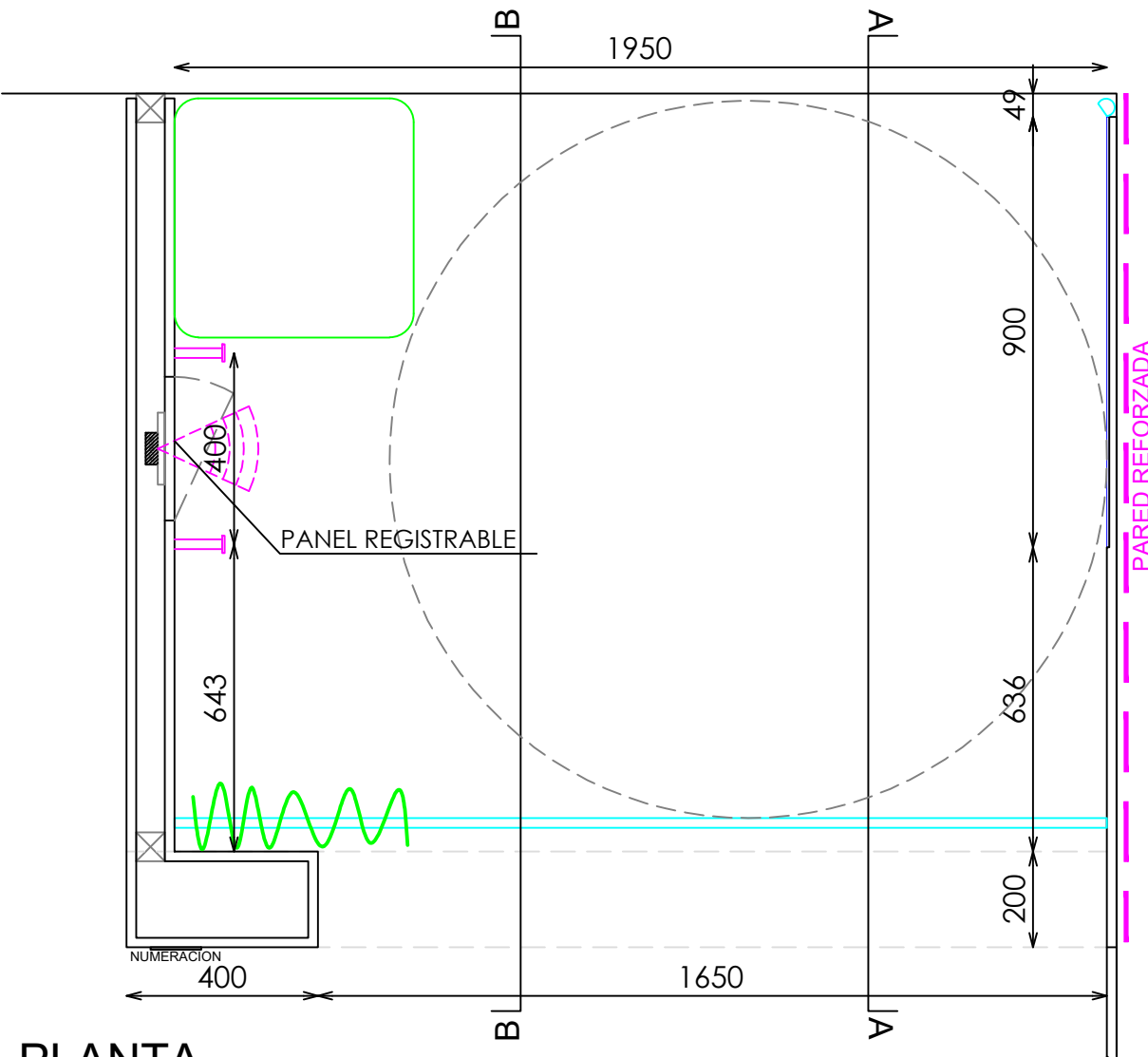
PLANTA
