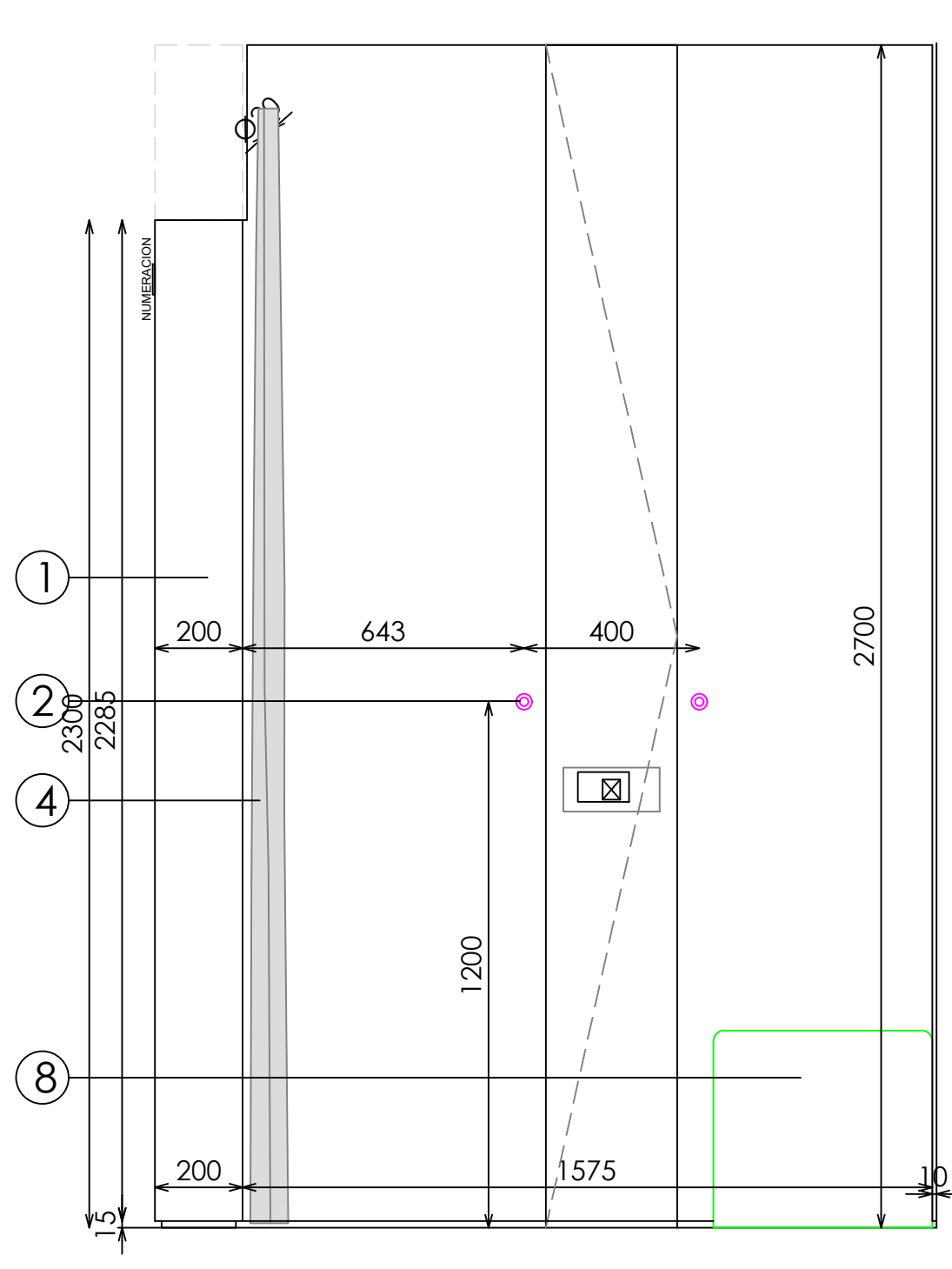
ALZADO LATERAL CUELGA
