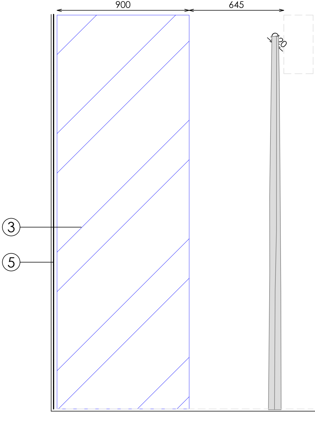
ALZADO LATERAL ESPEJO
